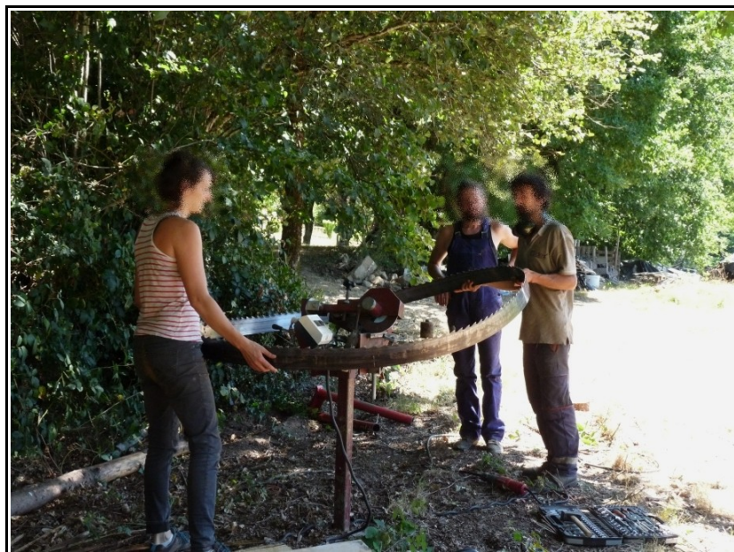
L'affûtage de la lame
